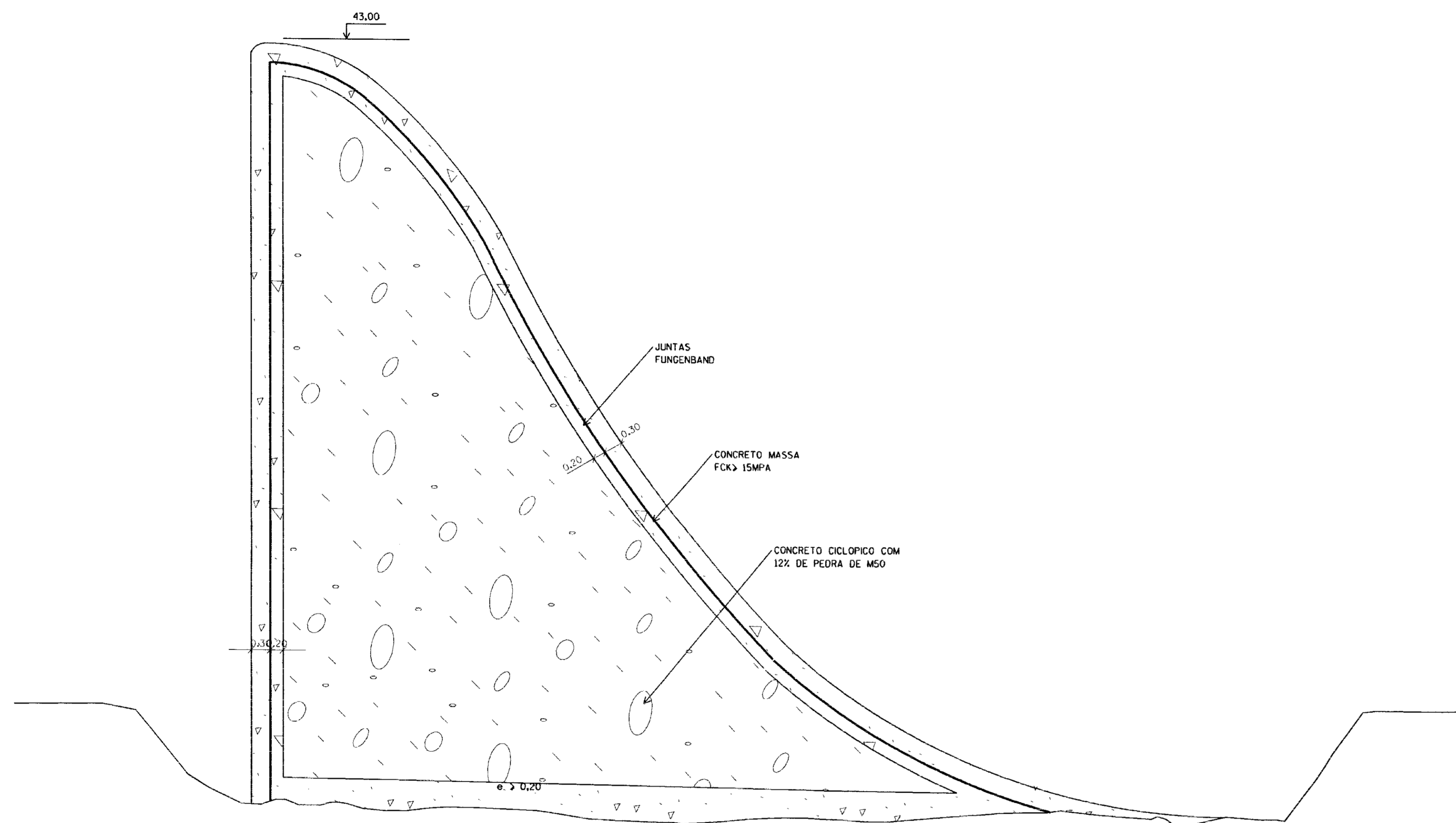
TRECHO SUBMERSÍVEL ESC. ——— 1:50
