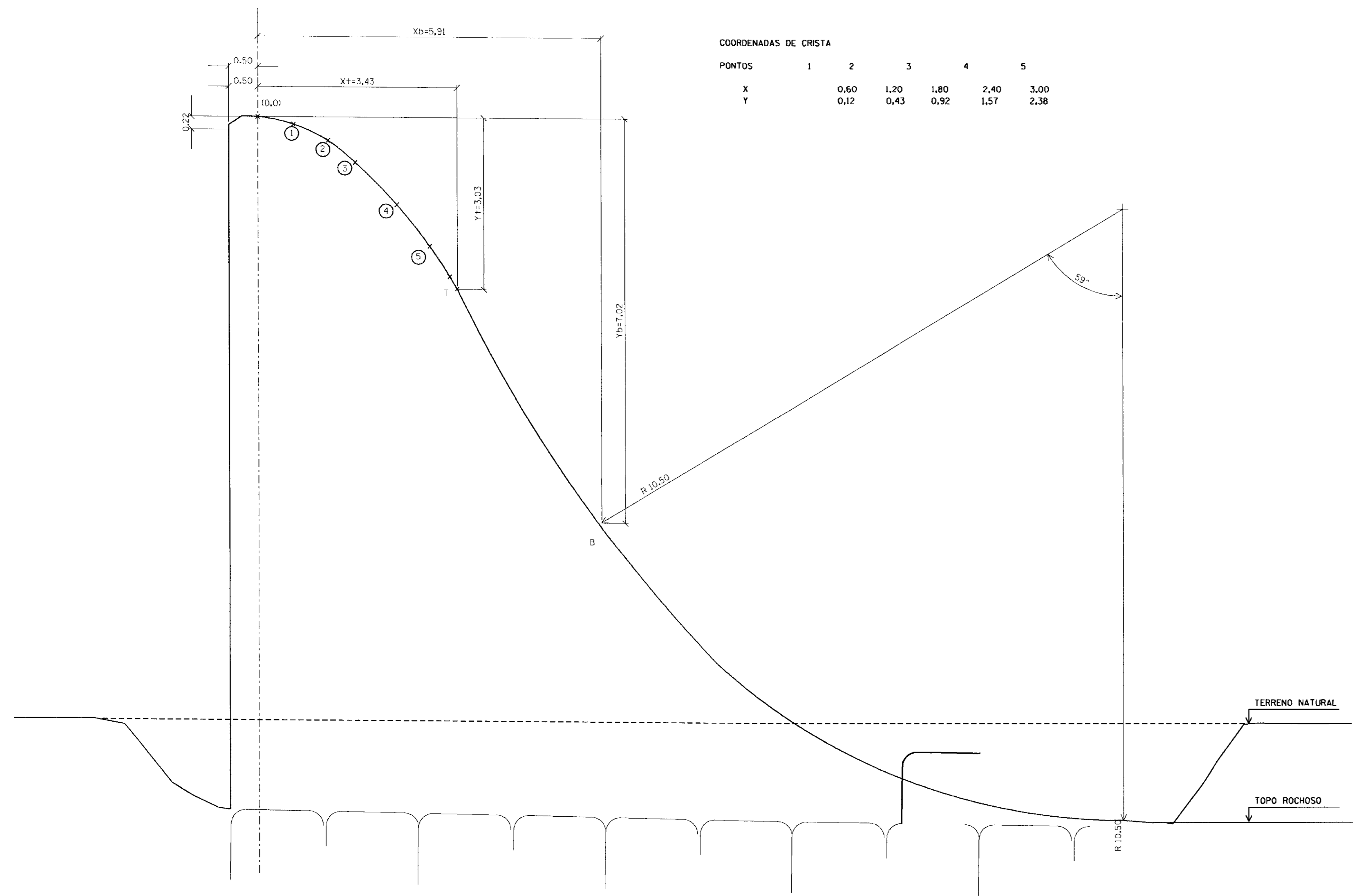
TRECHO SUBMERSÍVEL ESC. 1:50
