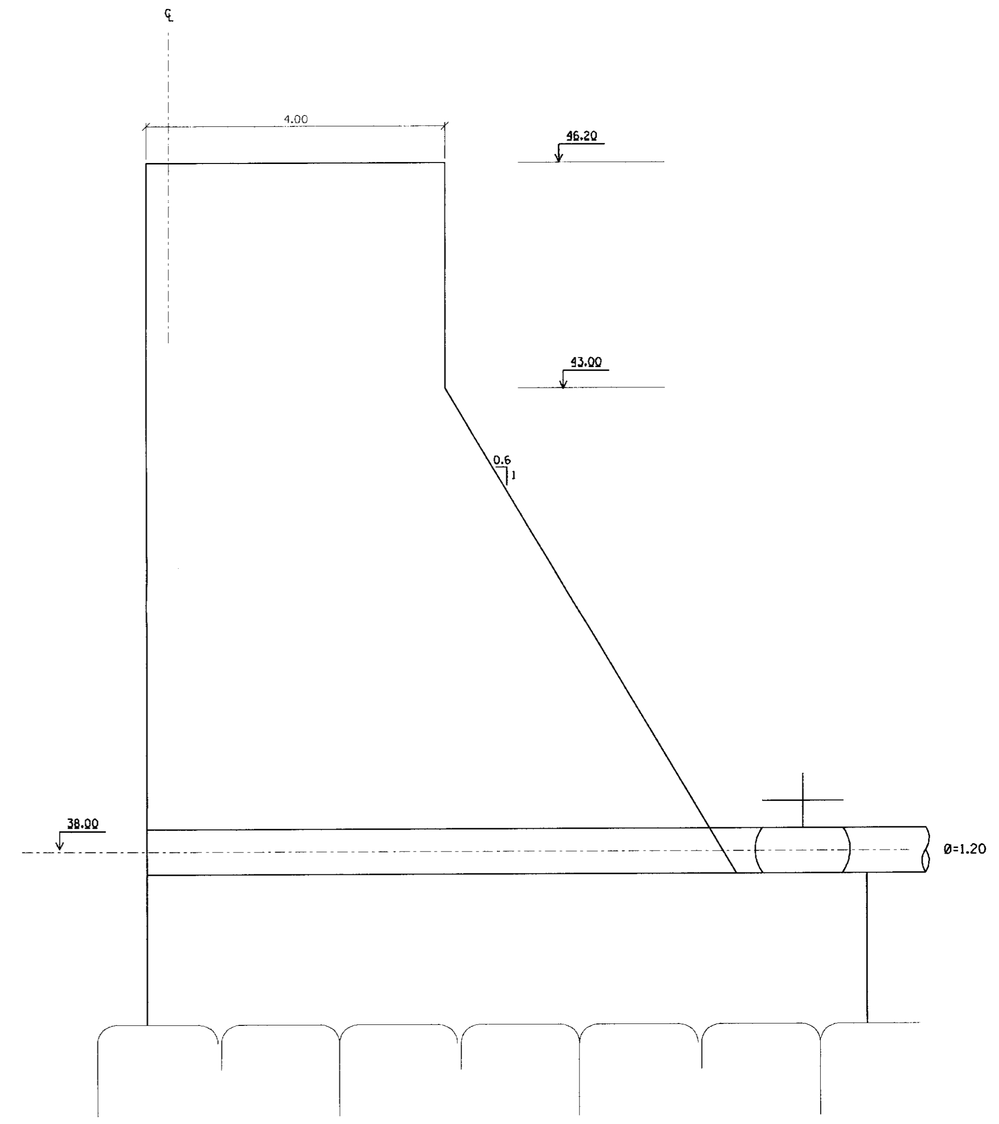
TOMADA D'ÁGUA (ESTACA 0 + 10) ESC. 1:50
